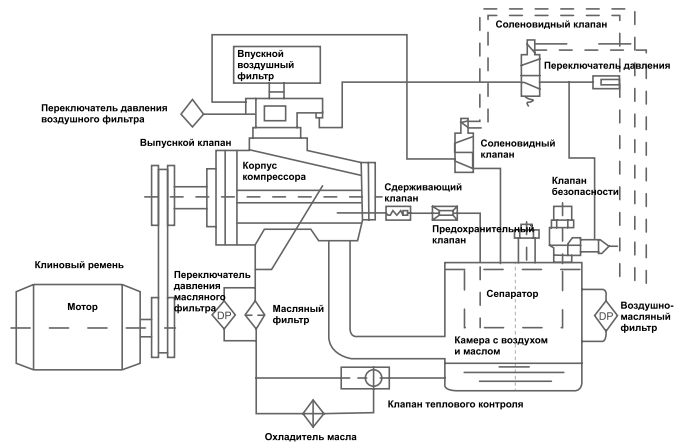
Схема технологического процесса (30 кВт)
