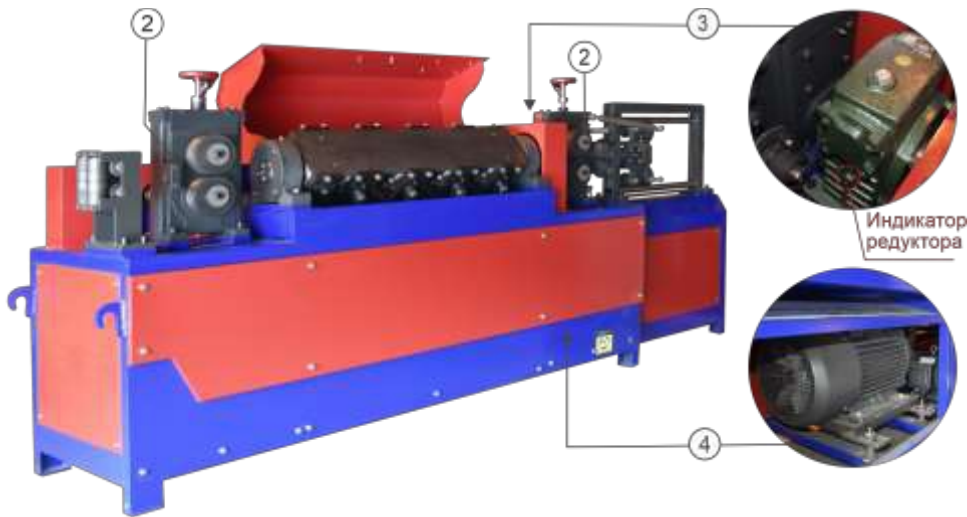
Рис. 2. Тяговая часть
